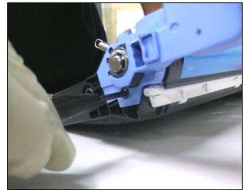
40. Para desmontar la unidad de cilindro primero sacar los tornillos de la manija azul del lado sin engranajes.
