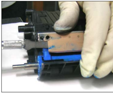
26. Antes de sacar la cuchilla cortar con un estilete el sello de espuma de goma.
