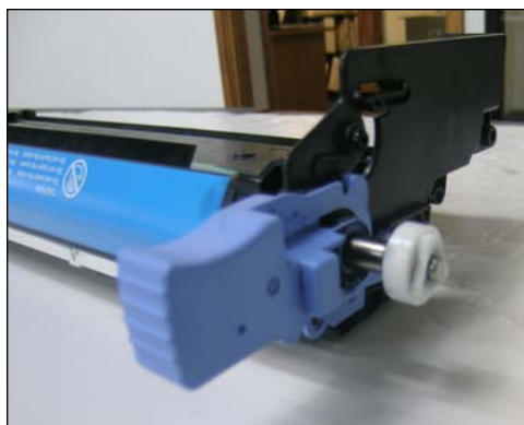
47. El eje se suelta desde el otro lado.
