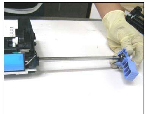
48. Deslizar el eje completamente hacia afuera.
