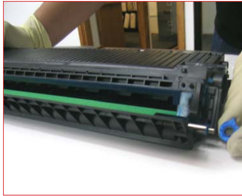
*EXTRACCION DEL RODILLO DE ALIMENTACIÓN 28. Sacar los dos sellos de felpa en cada extremo del rodillo.
