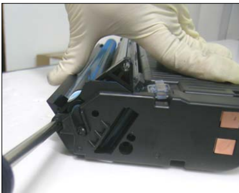
16. Sacar los dos tornillos de lado opuesto como se muestra.
