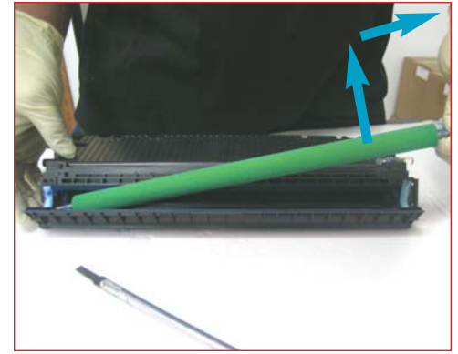
35. Levantar y deslizar hacia afuera el rodillo de alimentación como se muestra.
