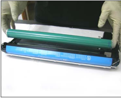
49. Sacar el cilindro como se muestra.
