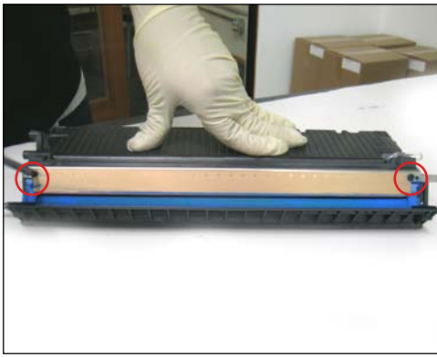
25. Sacar los dos tornillos que sujetan la cuchilla de dosificación.
