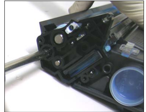
21. Ahora desmontar el soporte del rodillo sacando los dos tornillos como se muestra.
