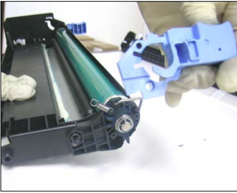
41. Soltar la manija de su clip y sacar como se muestra.
