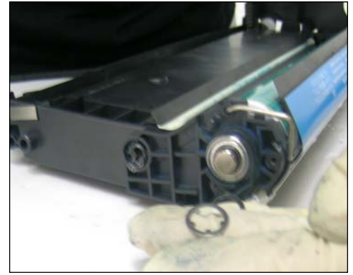
43. Sacar el aro de retención del cilindro.
